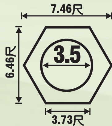
高16.1尺底座平面圖
