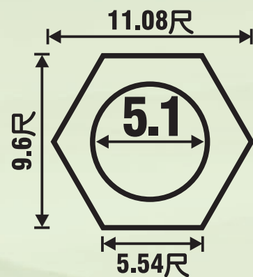
高26.2尺底座平面圖
