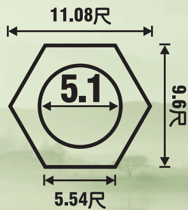
高31尺底座平面圖
