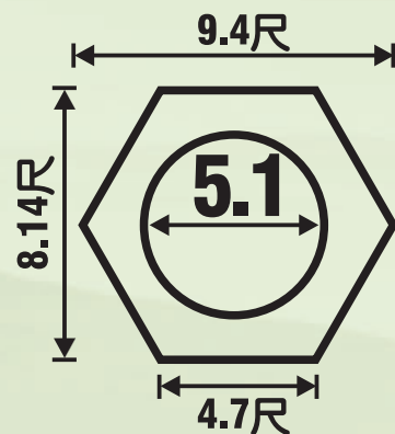
高21.8尺底座平面圖
