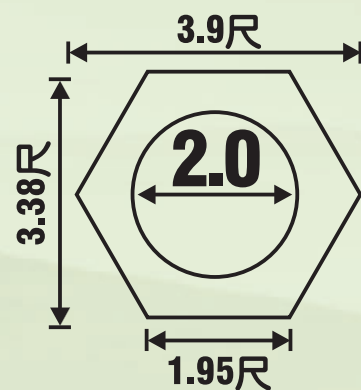
高6.5尺底座平面圖
